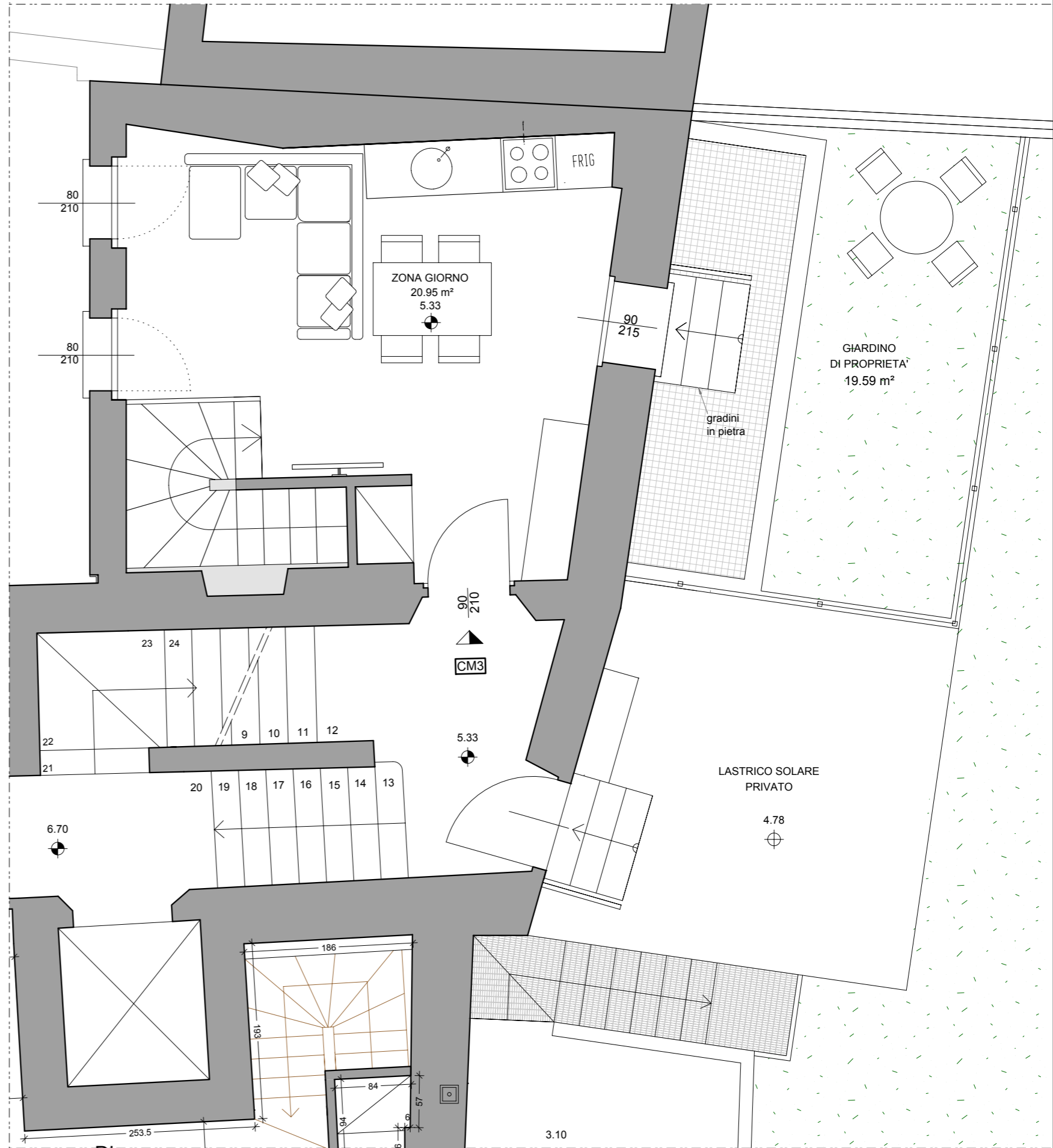
PLANIMETRIA PIANO SECONDO QUOTA +5.33
