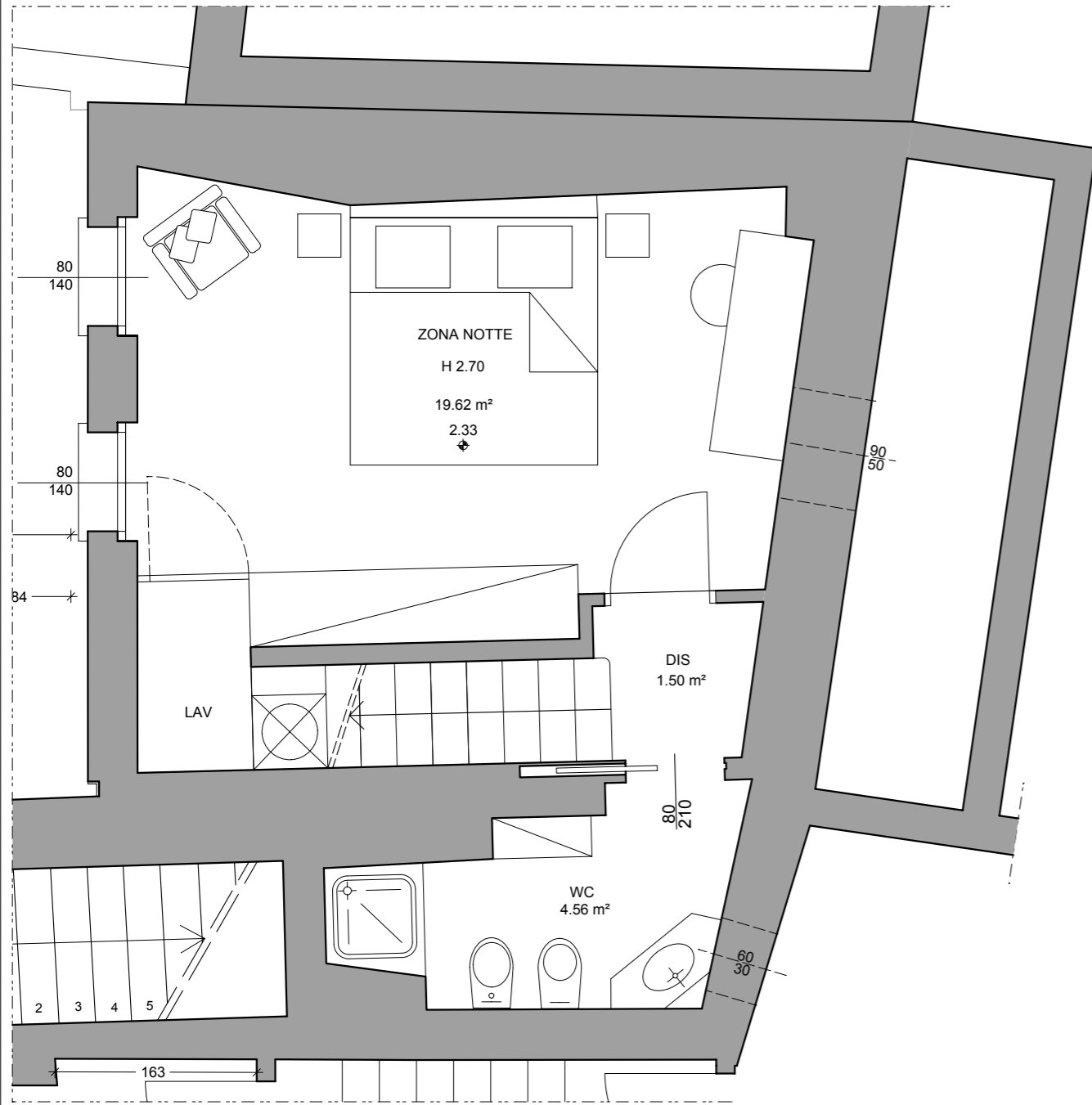
PLANIMETRIA PIANO PRIMO QUOTA +2.33
